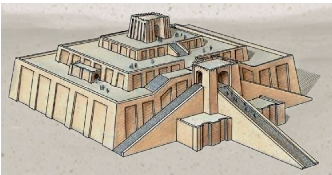
Zikkurat
